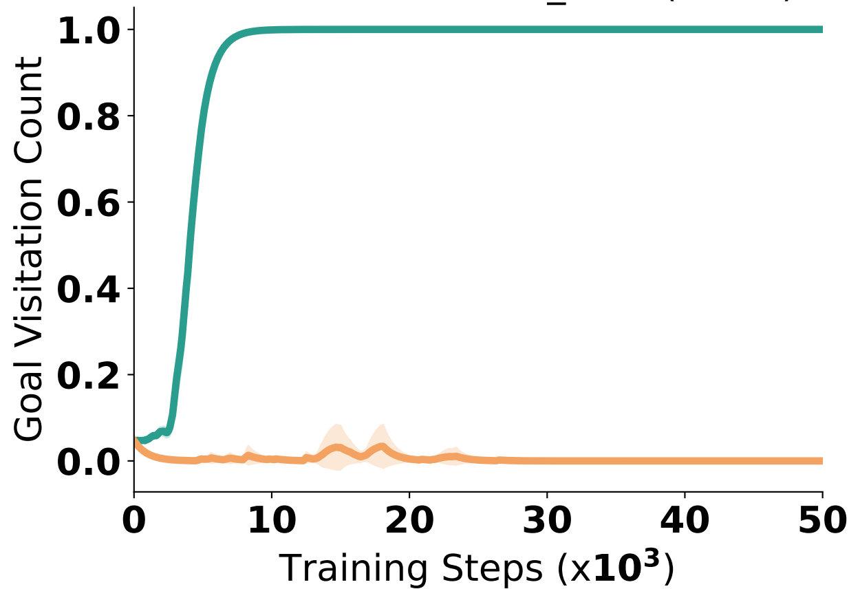
Gridworld-Bottleneck_Level(100%)
